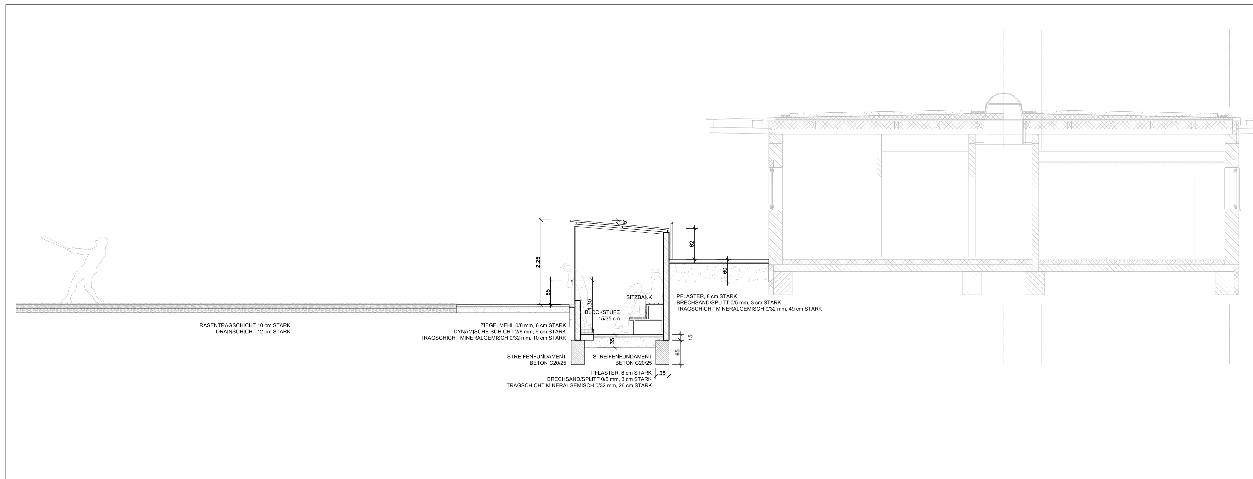
SCHNITT C-C M.1:50
