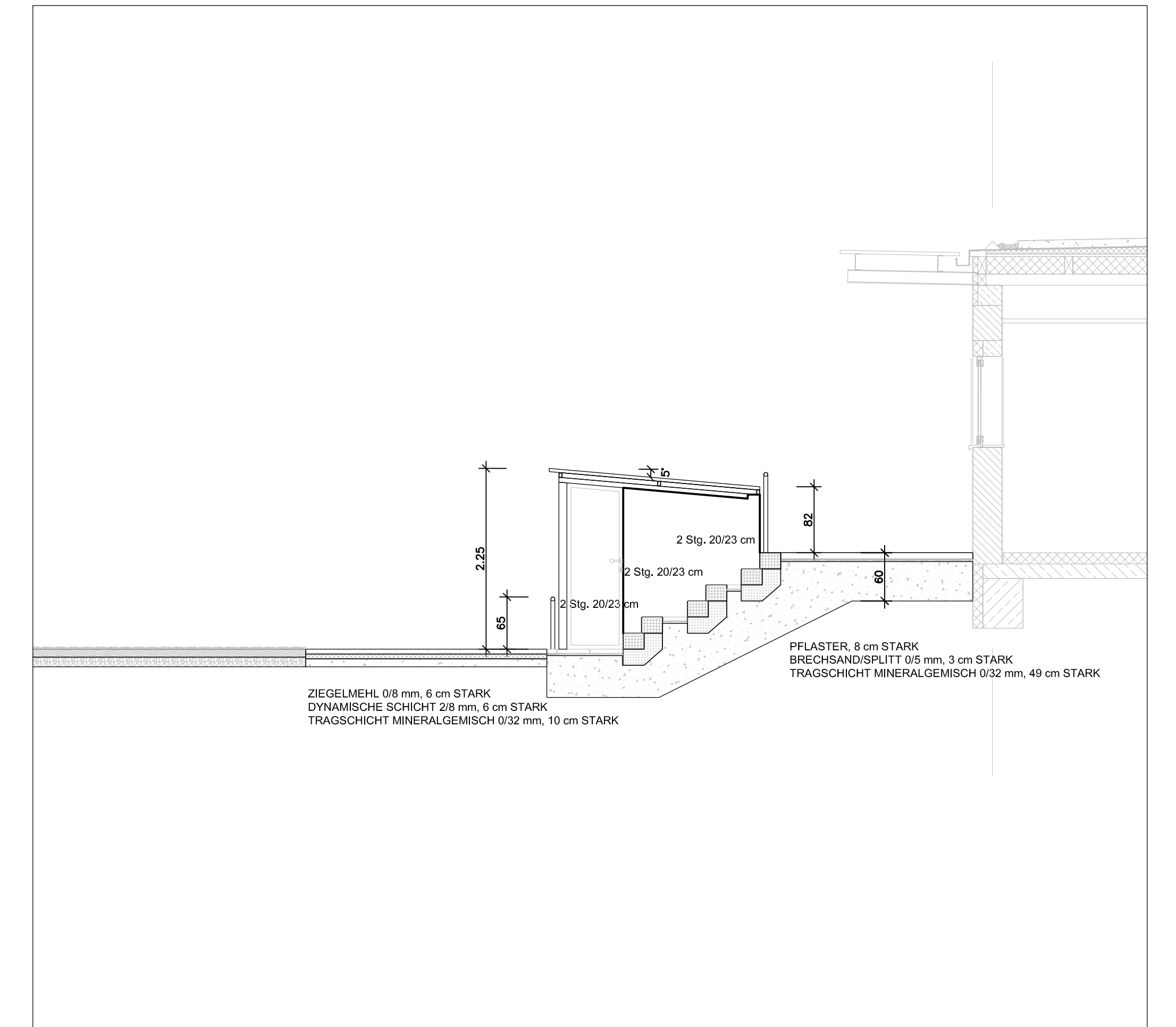
SCHNITT D-D M.1:50
