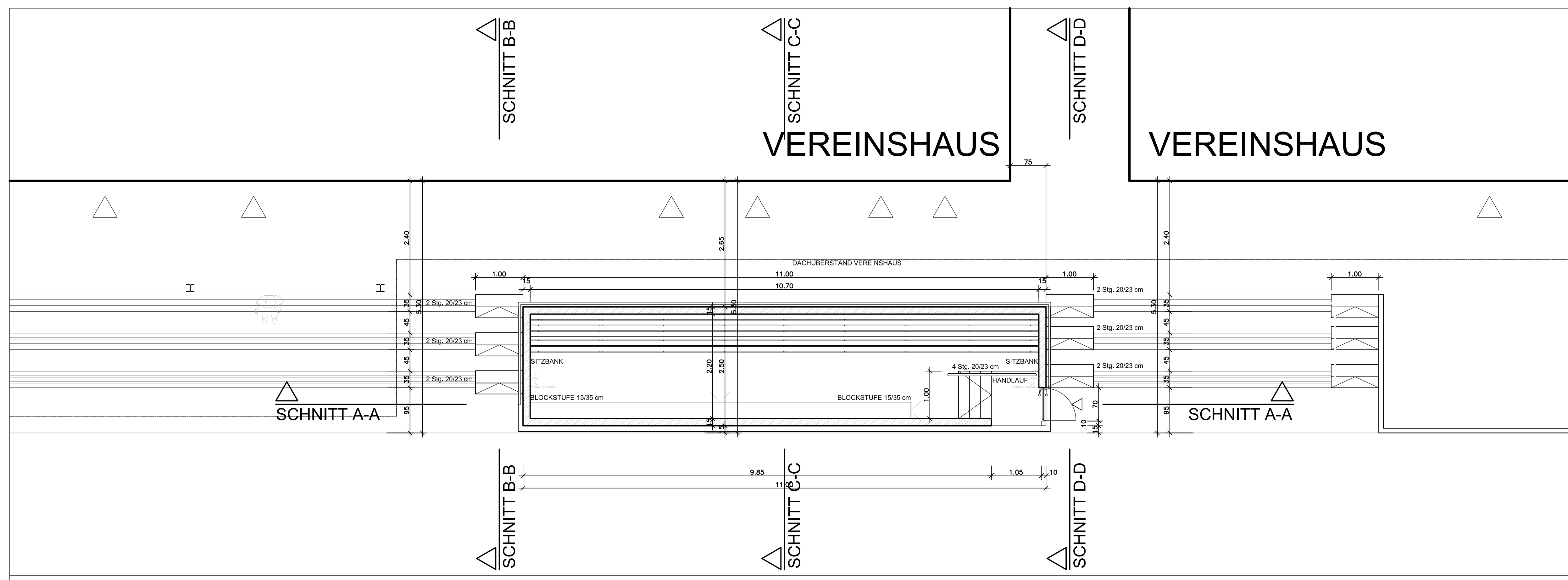
GRUNDRISS M.1:50
